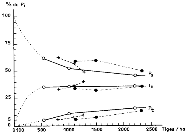
FIG. 6. — Influence de la densité sur l'interception ( I_n ), la pluie arrivant directement au sol ( P_s ) et l'écoulement le long des troncs ( P_t ) dans des plantations de Douglas. (0. nos résultats, + Mitscherlich et Moll 1970, ● Aussenac 1975).
